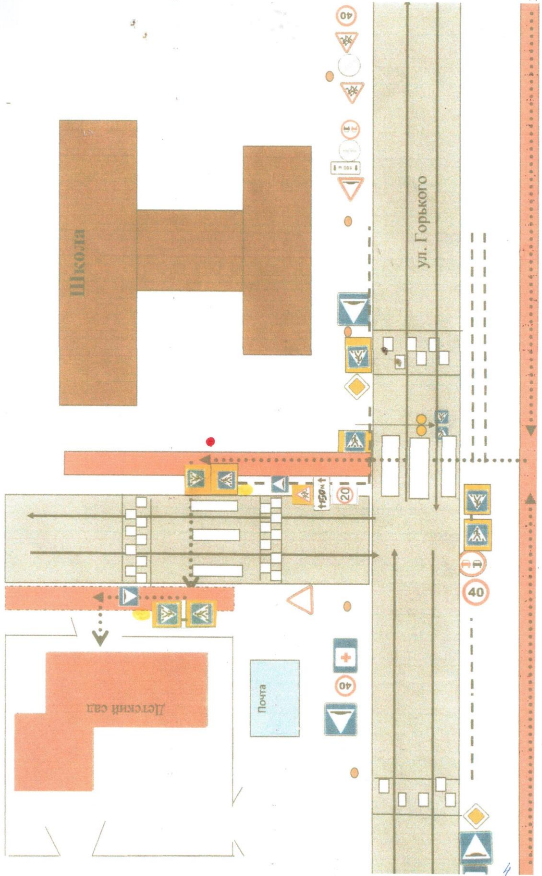
План - схема району розположення МБДОУ №18
